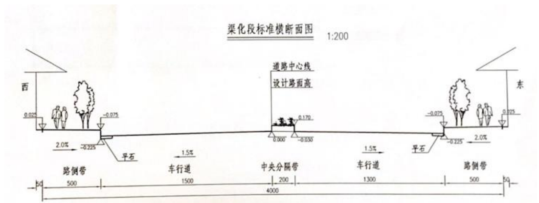
图 2-2 渠化段横断面设计图
