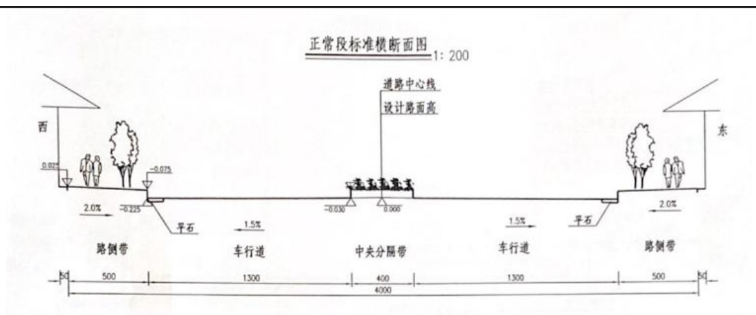
图 2-1 正常段横断面设计图
